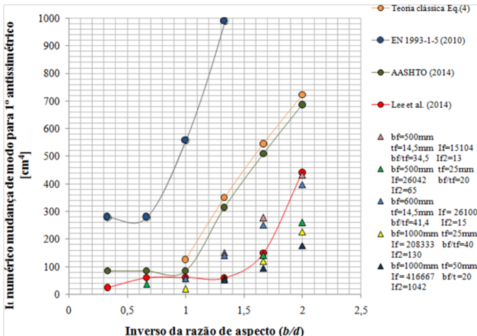
Figura 5 – Momento de inércia mínimo I_1 em função da esbelteza e da configuração geométrica das mesas.
