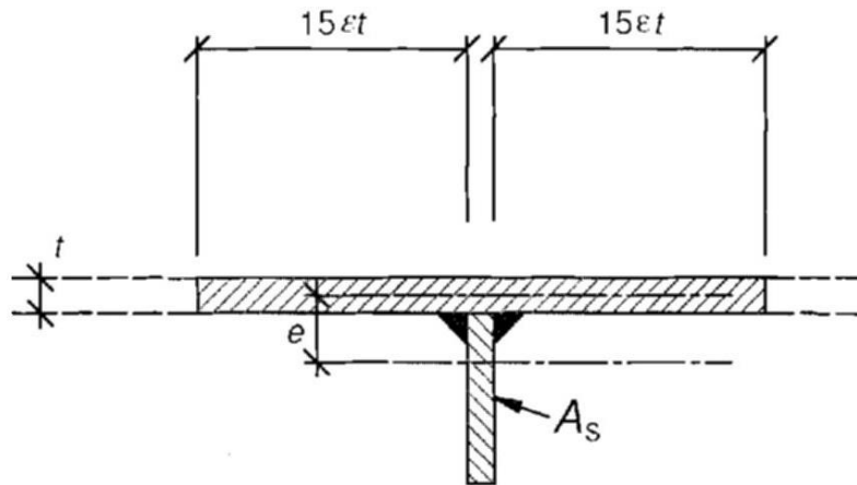
Figura 1 – Seção transversal efetiva de um enrijecedor intermediário.
