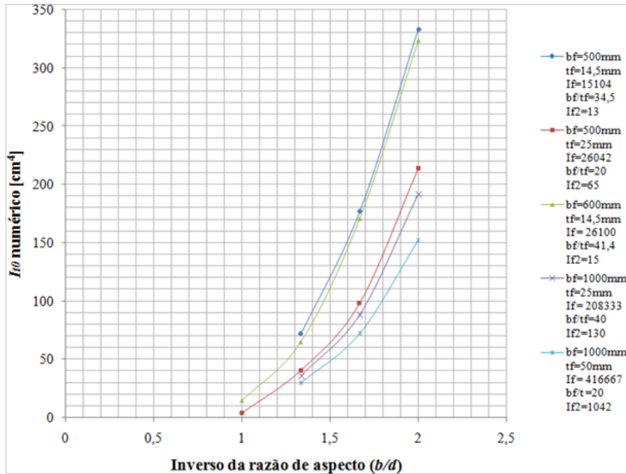
Figura 4 – Momento de inércia mínimo I_{10} em função da razão de aspecto e da configuração geométrica das mesas.
