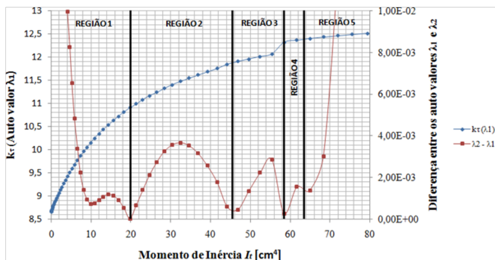
Figura 2 – Variação de k_r e variação da diferença entre \lambda_1 e \lambda_2 em função do momento de inércia do enrijecedor.
