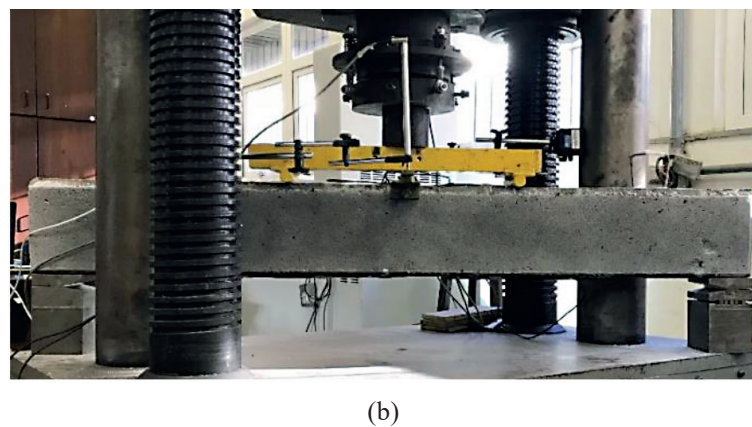
Figura 1 – (a) Detalhamento da viga, (b) ensaio Tirado (2022).
