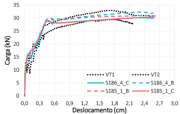
Figura 9 – Gráfico carga x deslocamento SOLID 185.
