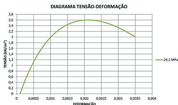
Figura 3 – Tensão x deformação específica código modelo ( fib , 2013)
