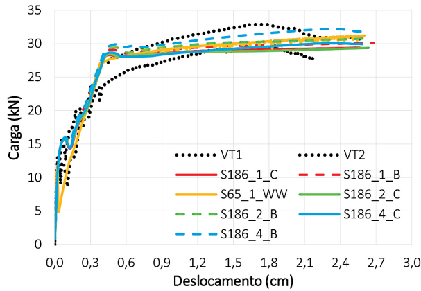
Figura 7 – Gráfico carga x deslocamento VT.
