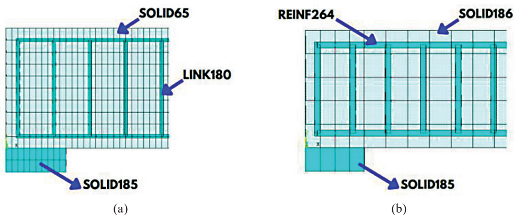
Figura 2 – Armadura (a) Discreta, (b) Incorporada.
