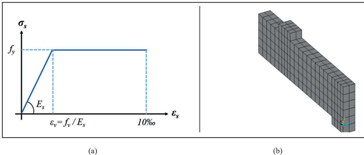
Figura 4 – (a) Tensão x deformação específica aço (LAZZARI, 2016); (b) eixos do modelo.
